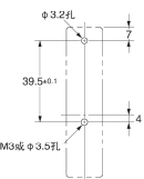
安装孔加工尺寸
