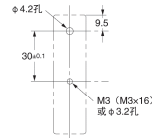
安装孔加工尺寸
