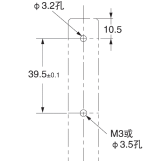
安装孔加工尺寸
